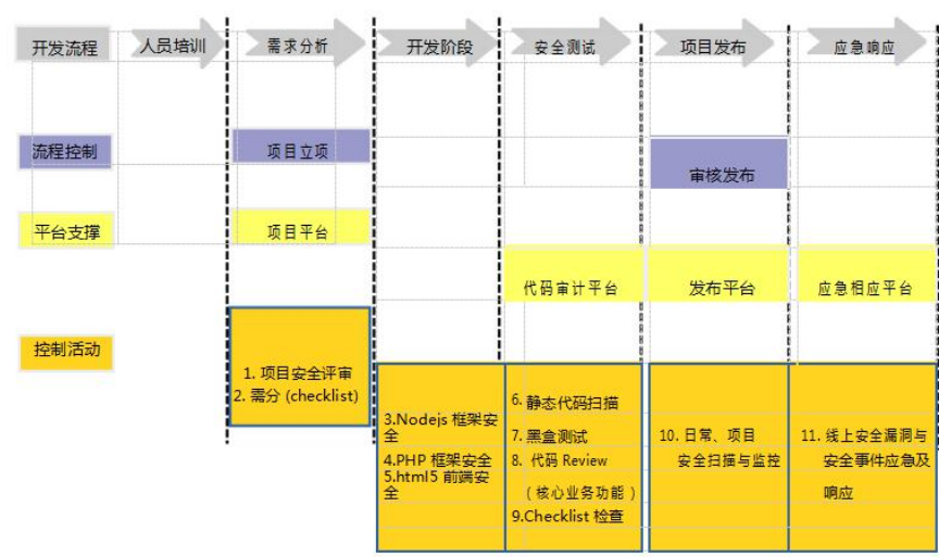
图 1 SDL 流程图
